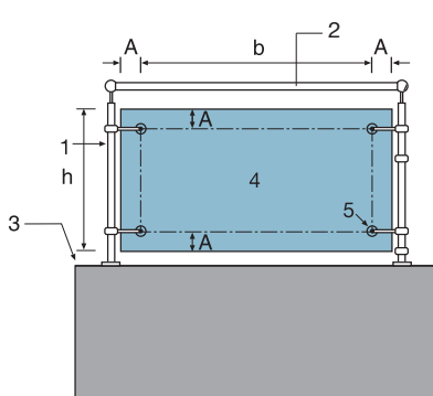
Figur 7a. Glas fastholdt med gennemgående punktbeslag/bolte.
